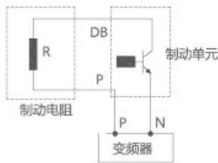
典型电路图
